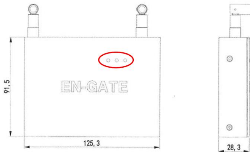
Figura 40 - Dimensioni dispositivo
