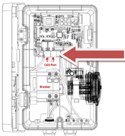
Figura 14 - Sistema di comunicazione
