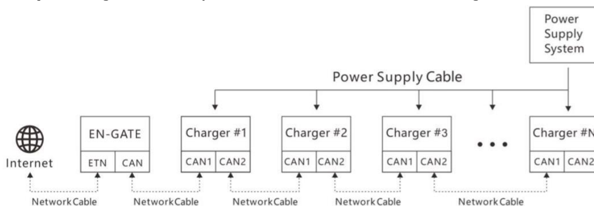
Figura 38 - Collegamento tra ZVM-GATEWAY e caricatori
