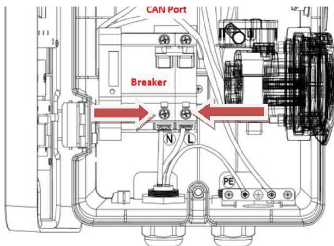
Figura 13 - Connessione dei cavi AC di uscita (2)
