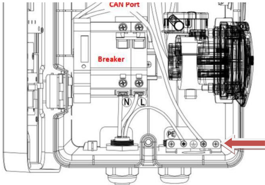
Figura 11 - Collegamento del terminale di terra
