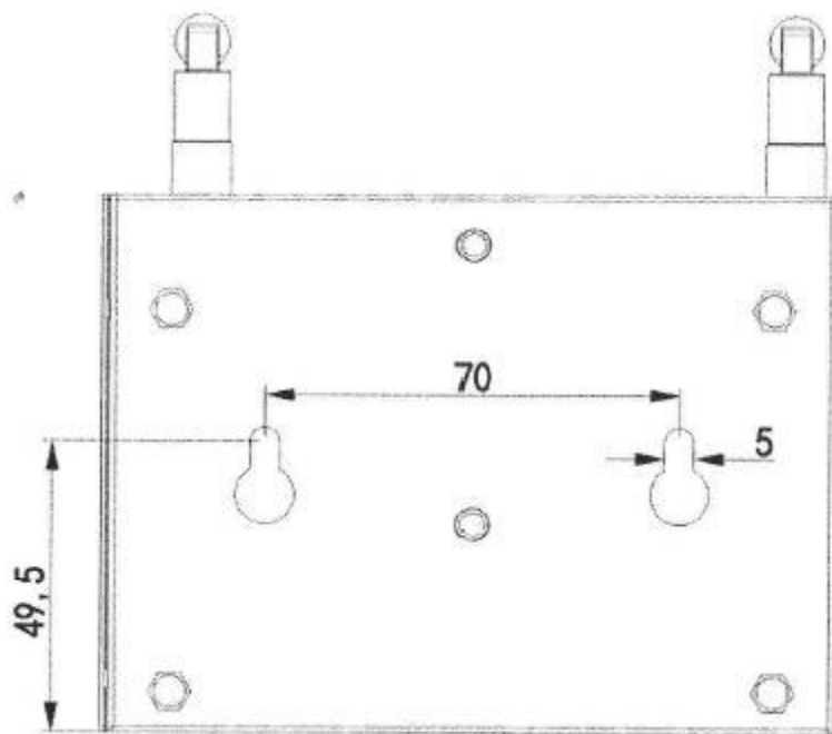
Figura 381 - Dimensioni per installazione
