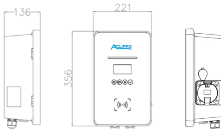
Figura 4 - Vista frontale, laterale della stazione di ricarica
