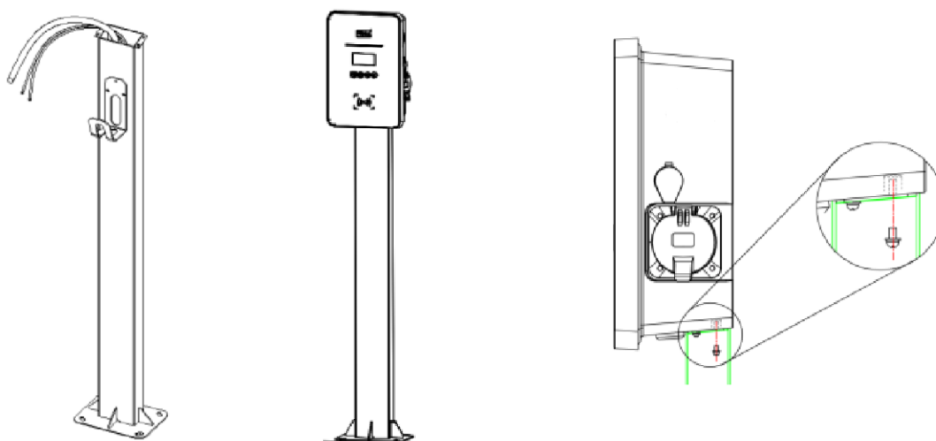
Figura 18 - Posizionamento pilone di supporto
