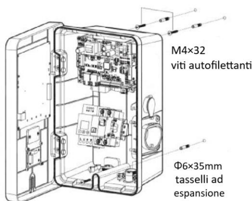
Figura 16 - Posizionamento viti per montaggio a parete
